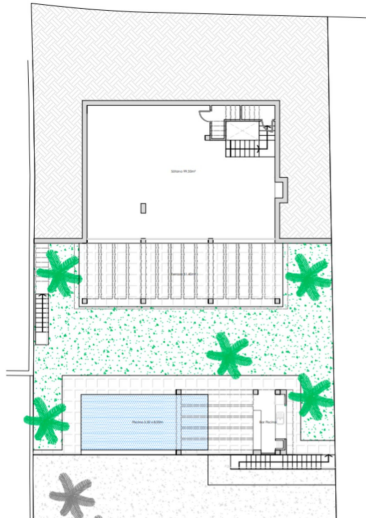
Planta Baja 1:125
