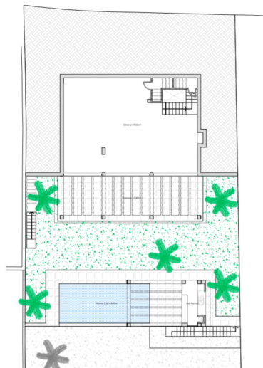
Planta Baja 1:125
